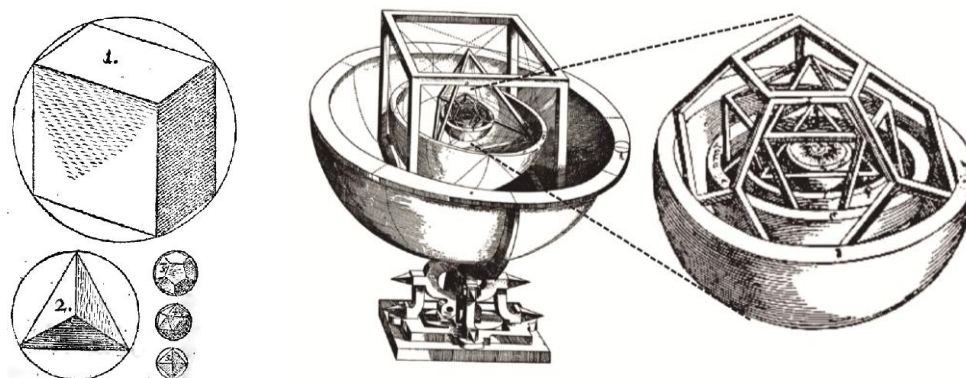
Figura 19. A la izquierda, los sólidos platónicos y los círculos que los circunscriben en KEPLER, 1619, V: 180; al centro, modelo del cosmos según el Mysterium Cosmographicum y detalle, a la derecha, de la esfera interior, con las órbitas de Marte, la Tierra Venus, Mercurio y el Sol en KEPLER, 1621: 24-25.
