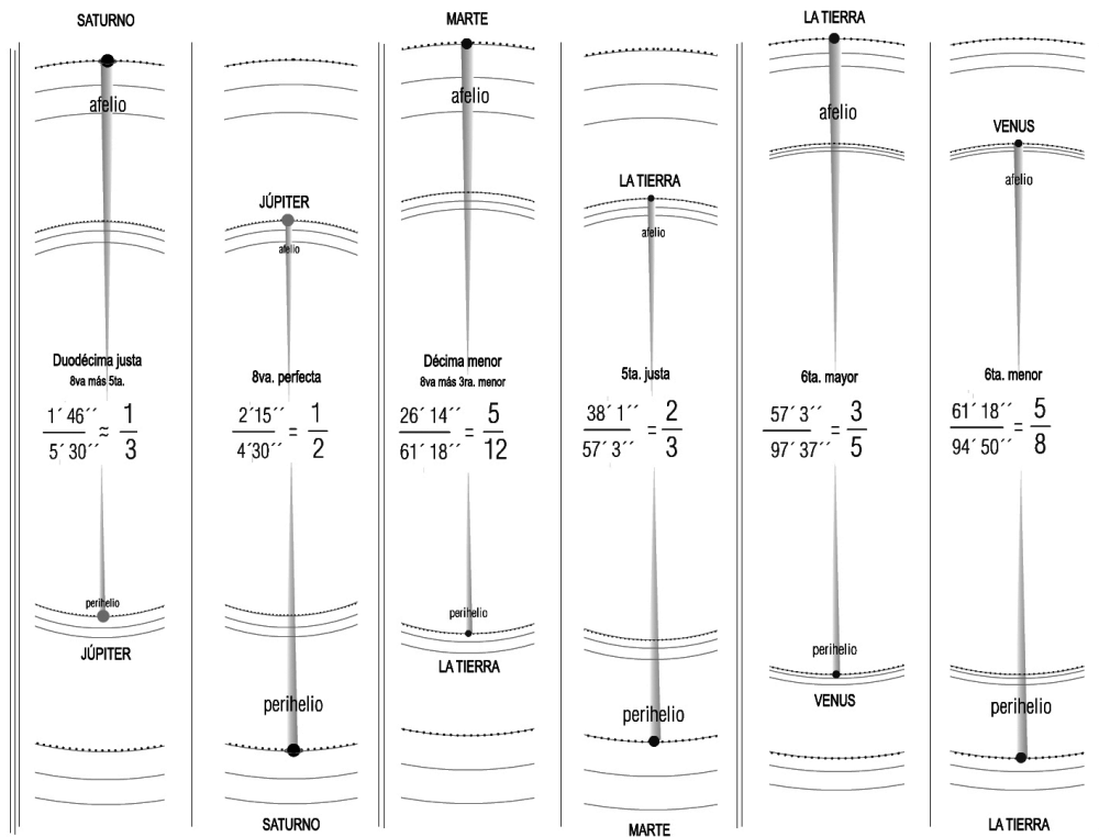
Figura 21. Armonía de los pares Saturno-Júpiter; Marte-La Tierra; La Tierra-Venus. Nótese la alternancia entre 6ta. mayor y menor que, a manera de dúo, “entonan” La Tierra y Venus.
